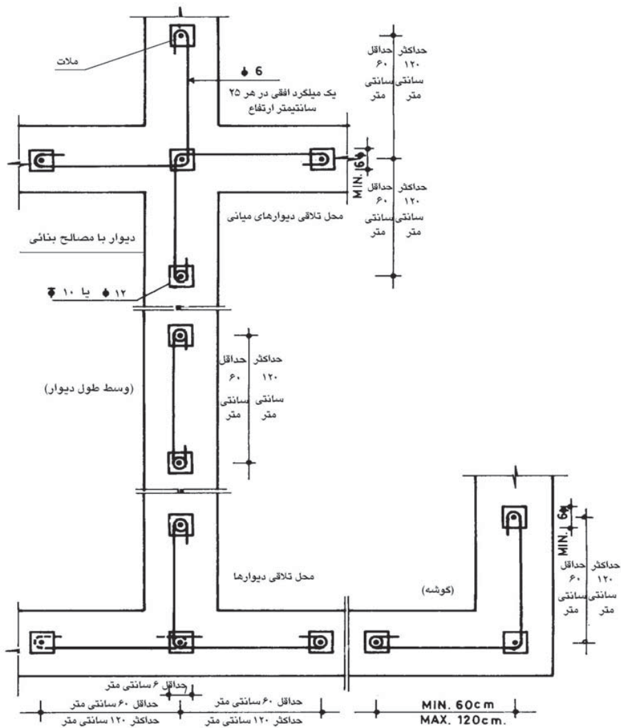
شکل (۸-۱-۱): جزئیات میلگردهای قائم و افقی مهاری دیوارها.
