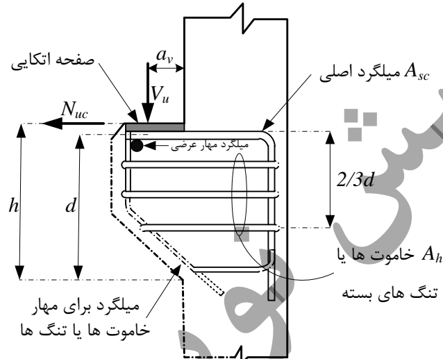
شکل ۹-۱۷-۲ میلگرد گذاری نشیمن
