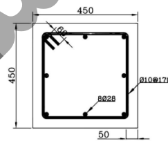
ستون 45-2.5
