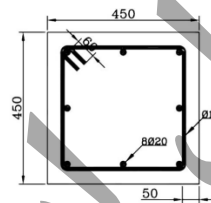
ستون 45-1.5
