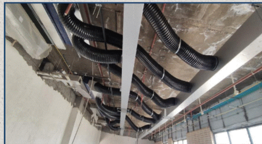
نصب لوله‌های فلکسیبل و پلنیوم باکس تهویه مطبوع طبقات
